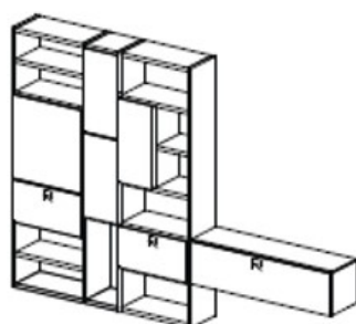
CM36 terra - pensile 2730x330x2272H
