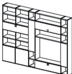
CM20 3030x330x2272H
