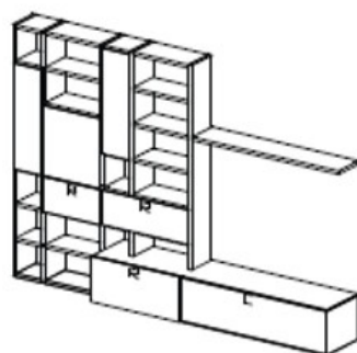
CM30 3330x500x2272H
